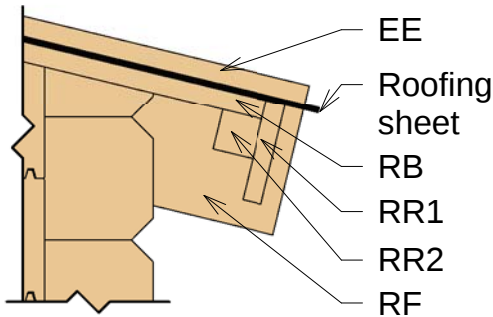
2) Facia
